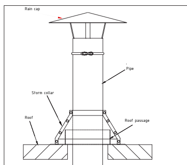
Aperçu d'installation en toiture
