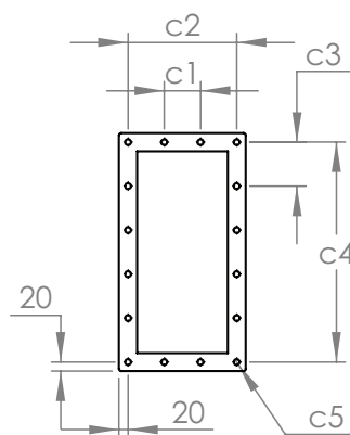
Vierkante inlaatflens
