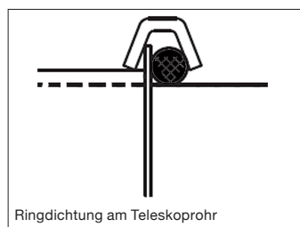
Ringdichtung am Teleskoprohr
