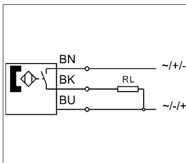
Sandariojo magnetinio jungiklio jungimo schema
