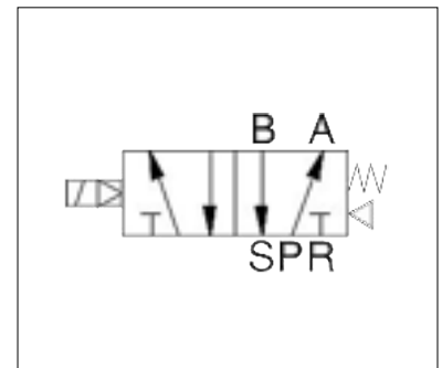
NAMUR solenoidinio vožtuvo sujungimo schema
