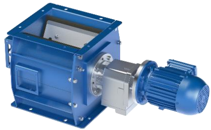
Zawory obrotowe
