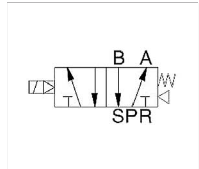
Bedradingsschema van de NAMUR magneetventiel
