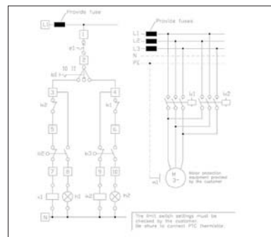
Bedradingsschema van elektrische actuator
