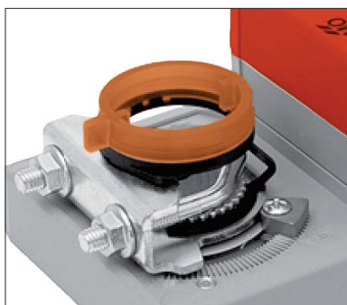
Visuele indicator gemonteerd op de vlinderklepas om positie aan te geven
