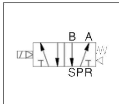
Bedradingsschema van NAMUR-magneetventiel
