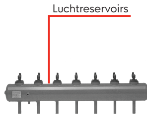
Luchtreservoirs
