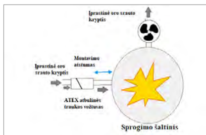
Paveikslas Nr.8 Srauto traukimas
