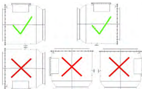
Paveikslas Nr.10 Montavimo kryptis
