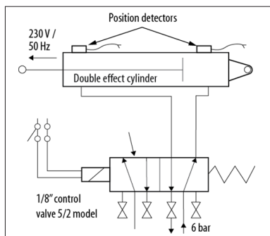
Aansluiting van lineaire pneumatische cilinder op pneumatische schuifkleppen van diameter Ø 80 t/m Ø 160 mm.
