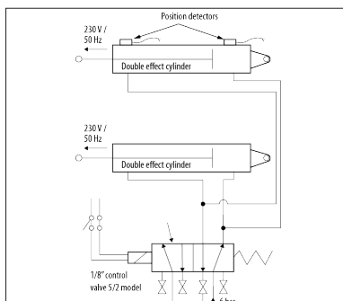
Aansluiting van twee lineaire pneumatische cilinders op pneumatische schuifkleppen vanaf diameter Ø 180 mm.
