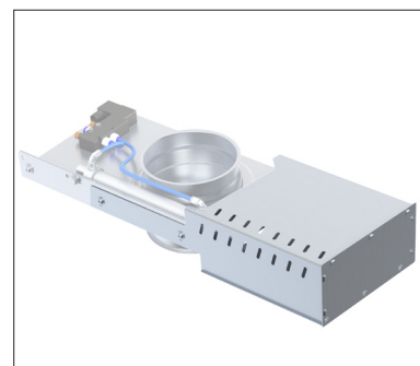
Schuifklep met beschermkap optie.
