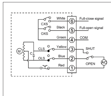
220 V AC pavaros elektros prijungimo schema
