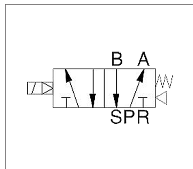
NAMUR elektromagnetinio vožtuvo prijungimo schema
