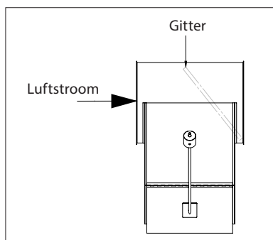
Luftstromrichtung (mit optionalem Gitter)
