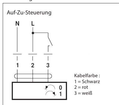
Schaltplan des elektrischen Antriebs
