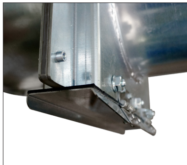
Entleerungsdeckel an der Unterseite der Klappe
