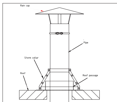
Proper installatie van een regenrok
