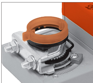
Visuele indicator gemonteerd op de vlinderklepas om positie aan te geven
