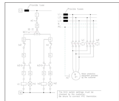
Bedradingsschema van elektrische actuator
