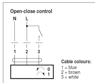
Bedradingsschema van een elektrische actuator
