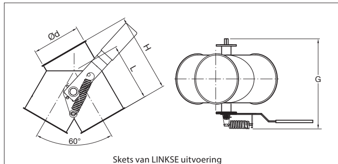
Skets van LINKSE uitvoering
