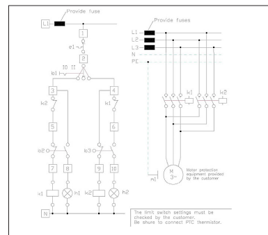
Bedradingschema van elektrische actuator
