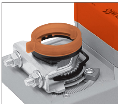
Visuele indicator gemonteerd op de vlinderklep om positie aan te geven
