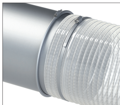
Exemple d'assemblage
